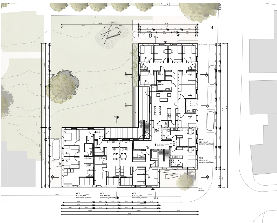
2. Obergeschoss
