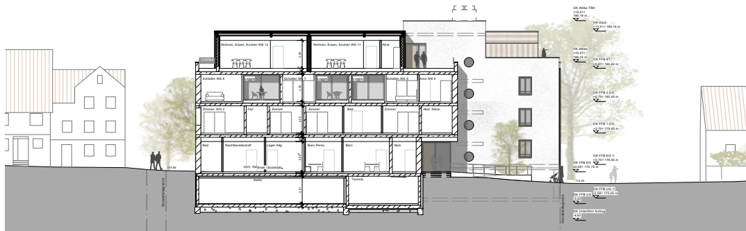
Schnitt B-B
