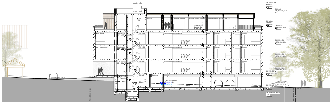
Schnitt A-A
