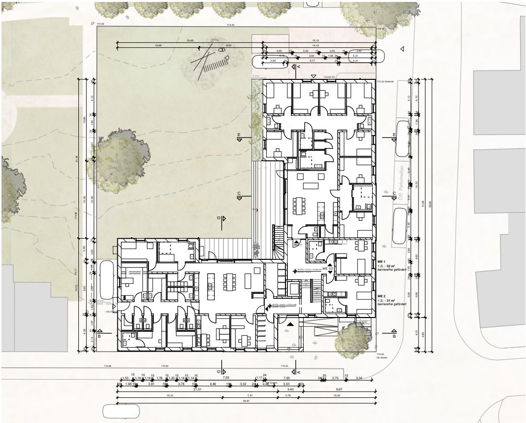
Erdgeschoss
