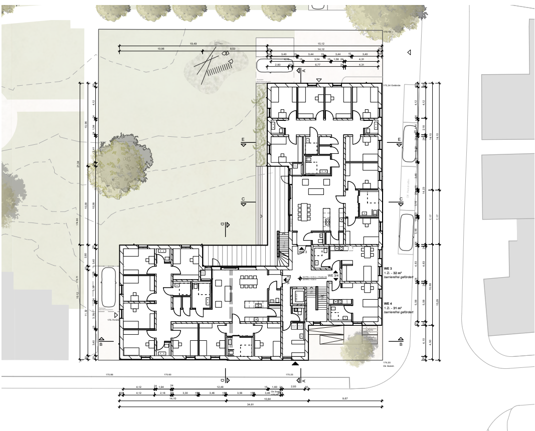
1. Obergeschoss
