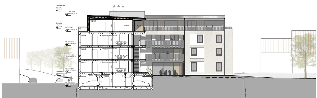
Schnitt C-C
