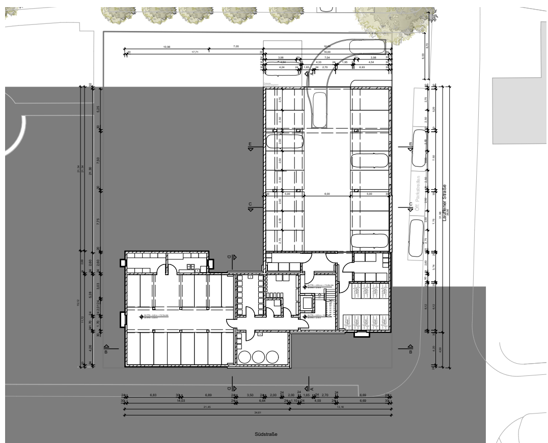
Untergeschoss
